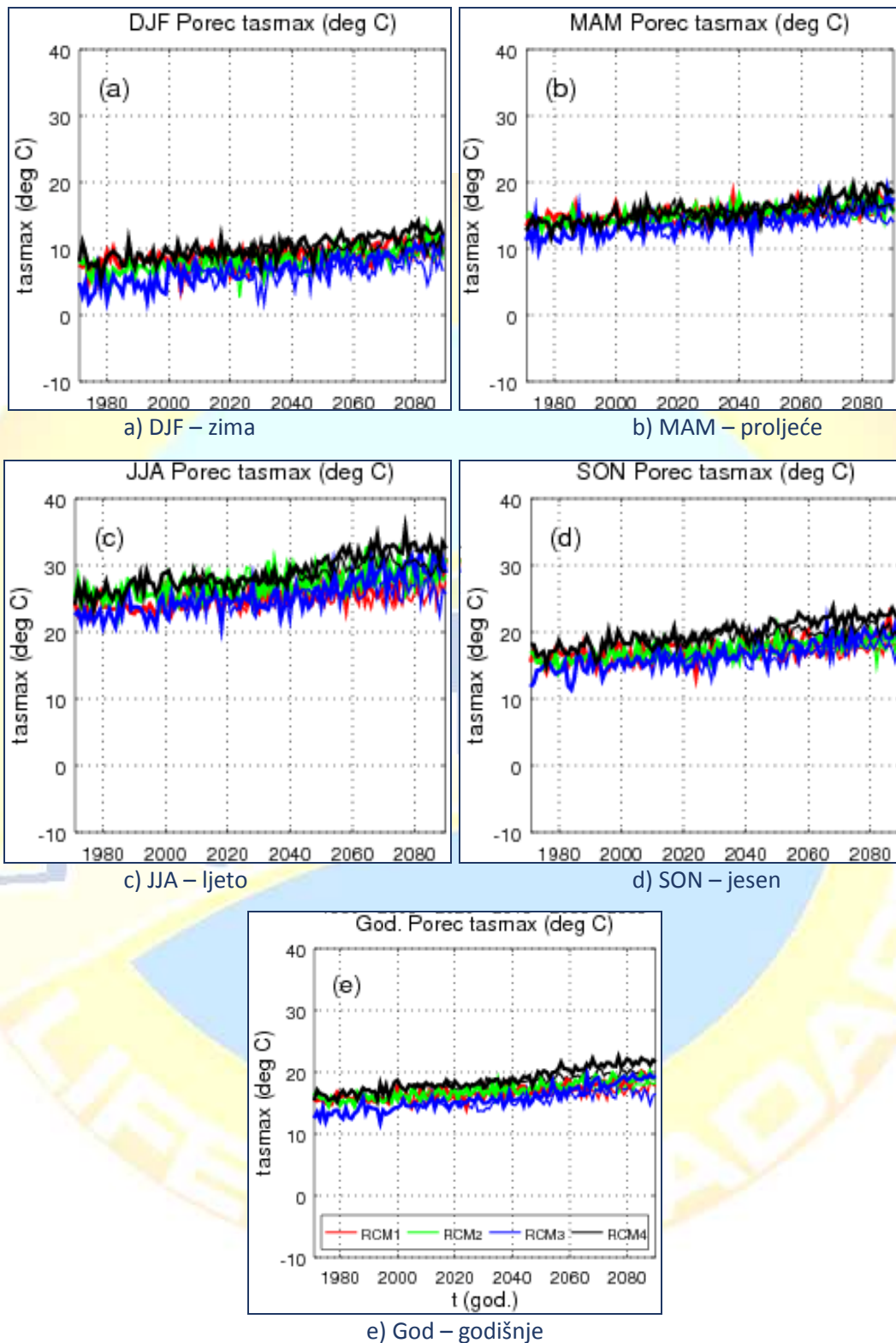
Slika 23. a) do e) Vremenski niz srednje sezone (DJF-zima, MAM-proljeće, JJA-ljeto, SON-jesen) i godišnje (God) srednje maksimalne dnevne temperature zraka za klimatološku postaju Poreč, za razdoblje 1971. - 2090. prema dva scenarija (RCP4.5 i RCP8.5) i četiri MedCORDEX regionalna klimatska modela (RCM1: GUF-CCLM4-8-18 (GCM: MPI-ESM-LR); RCM2: CNRM-ALADIN5.2 (GCM: CNRM-CM5); RCM3: CMCC-CCLM4-8-19 (GCM: CMCC-CM); RCM4: LMD-LMDZ4-NEMOMED8 (GCM: IPSL-CM5A-MR)). Mjerne jedinice: °C. Lokacija: Poreč.
